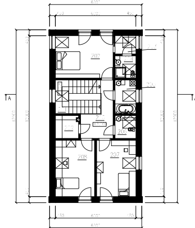
2. NADZEMNÍ PODLAŽÍ
