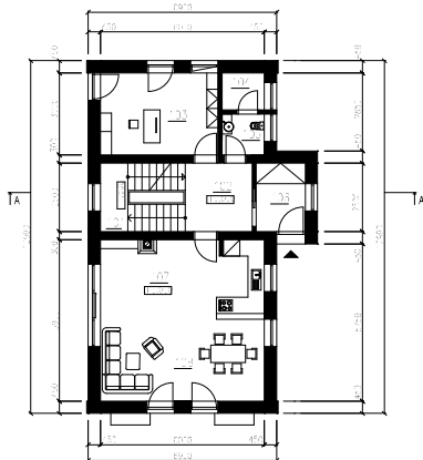
1. NADZEMNÍ PODLAŽÍ
