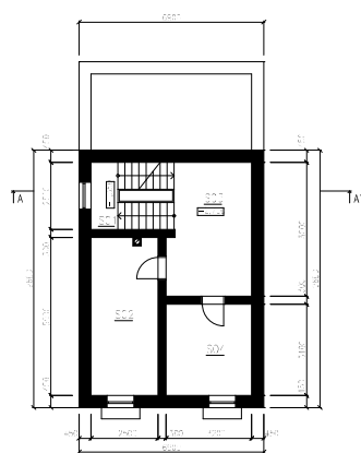
SUTERÉN:
